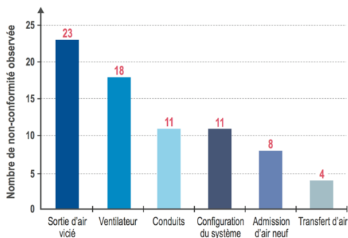
Figure 2. Non-conformités observées lors des diagnostics visuels de ventilation des 21 maisons de la campagne.
